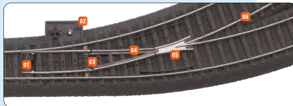
01 Aghi del deviatoio in pressofusione, impernati singolarmente 02 Struttura muraria fedele al prototipo nel meccanismo di posizionamento 03 Presa di contatto continuata dagli aghi sino all'elemento del cuore 04 Controrotaie di materiale del profilato 05 Elemento del cuore incorporato di metallo 06 Curva del deviatoio quale sezione di intersezione da 30°, raggio 360 mm
